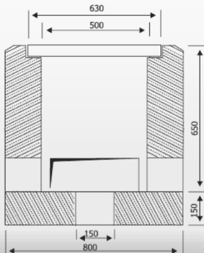
Przekrój poprzeczny
