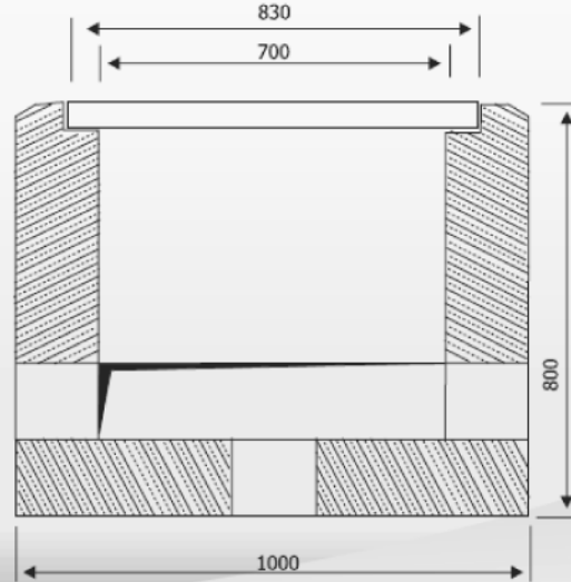
Przekrój podłużny
